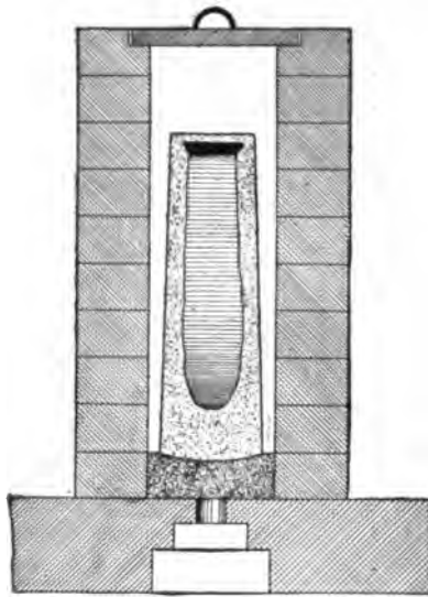
Fig. 112. Gjers Soaking Pit.
